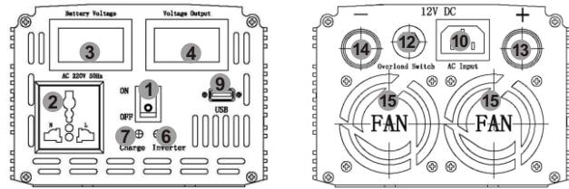
BEU2000L/3000L UPS逆变器面板
