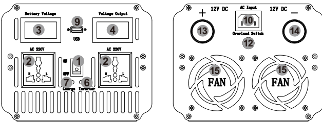
BEU5000L UPS逆变器面板
